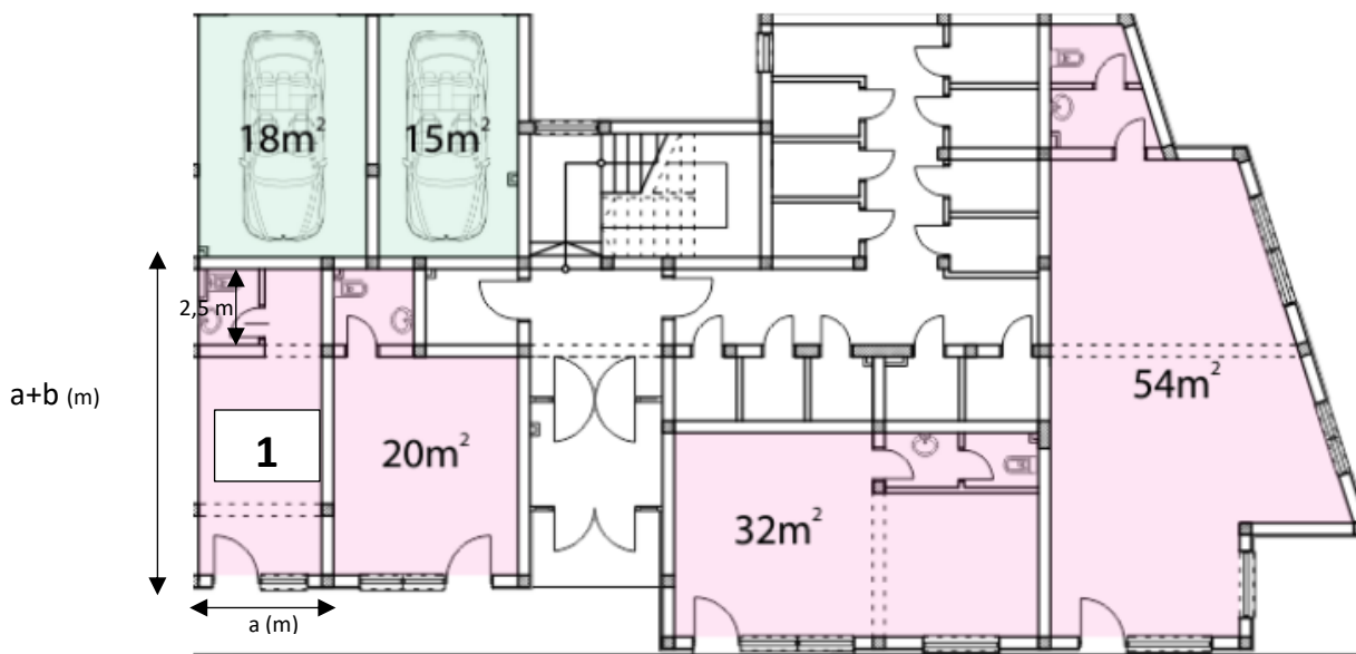
Slika broj 1: Osnova prizemlja (a=broj slova u imenu; b=broj slova u prezimenu; dimenzije svih otvora širina=1,00m+a cm; visina=1,95m +b cm).
